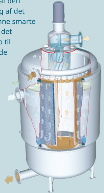
Illustration af varmeveksleren som er en central del af teknologien bag ENVOTHERM anlægget.
